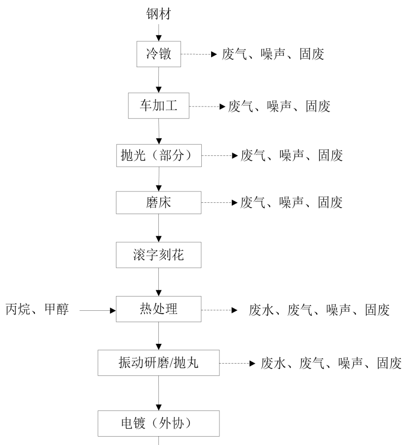
图 2.2-1 本项目五金配件生产工艺流程图
